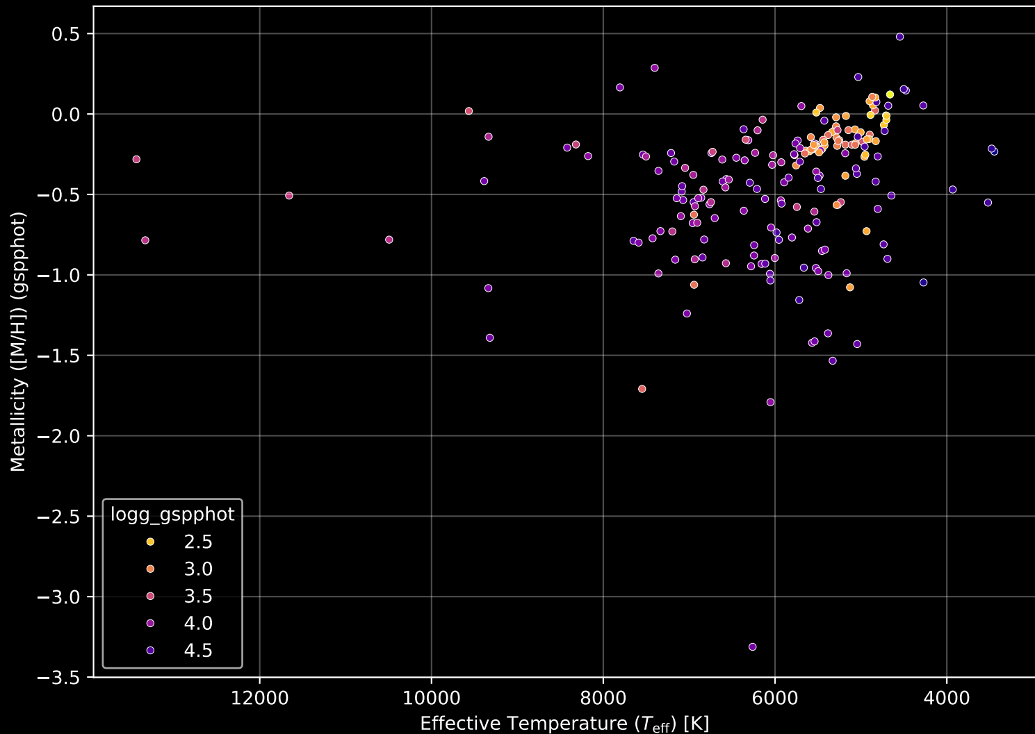
APOGEE DR17 Field: [K2_C13_178-11_btx] Stellar Population Parameters (n= 208)
